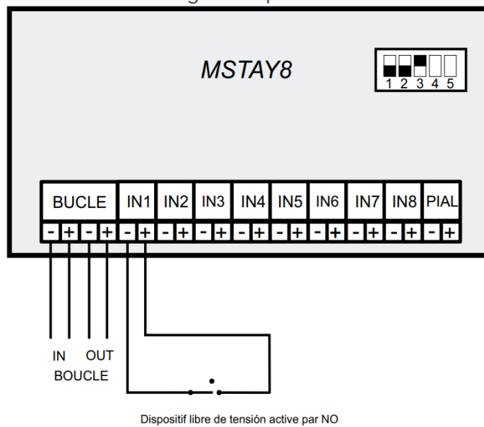
Figura 10. Schéma de raccordement MSATY8
