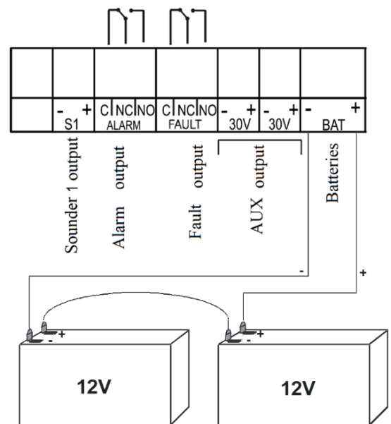
Figure 23. Schéma de raccordement des batteries
