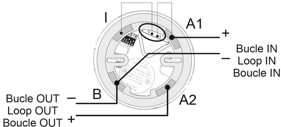
Figure 14A. Schéma de raccordement A50XZSDDR/A50XZSLDR
