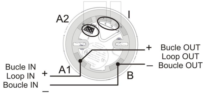
Figure 14D. Schéma de raccordement A30XZSDDR/A30XZSLDR
