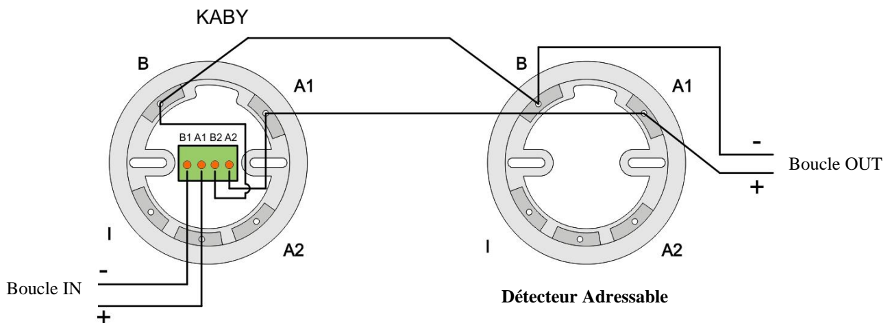
Figure 11. Schéma de raccordement KABY
