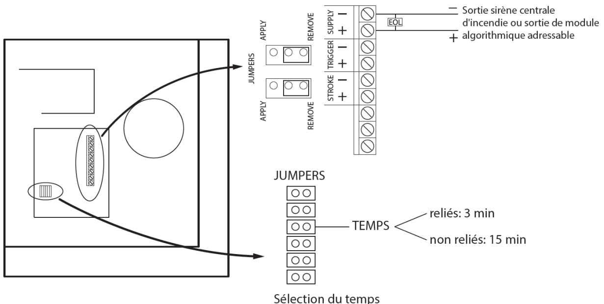
Figura 28 Schéma de raccordement CAEC
