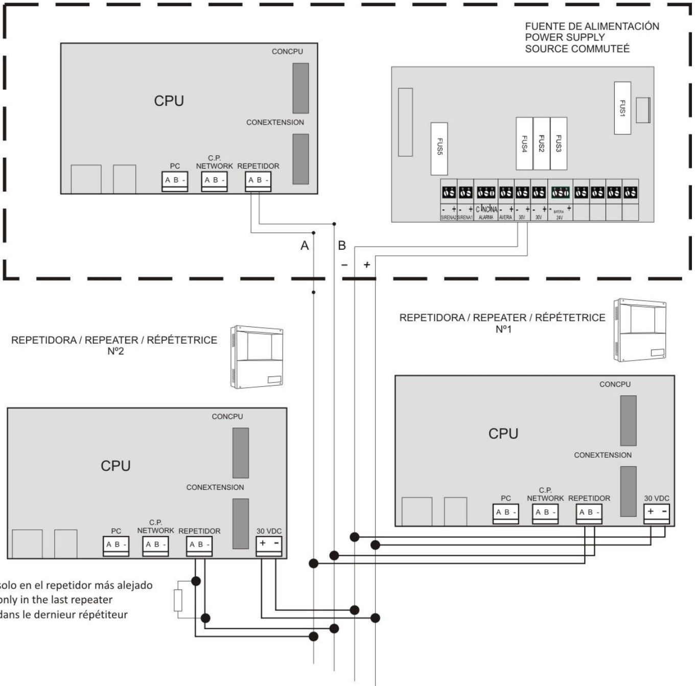
Figure 11. Raccordement des répéteurs
