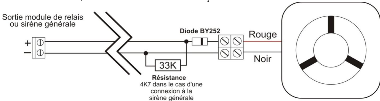
Figure 27. Schéma de raccordement SIR24F
