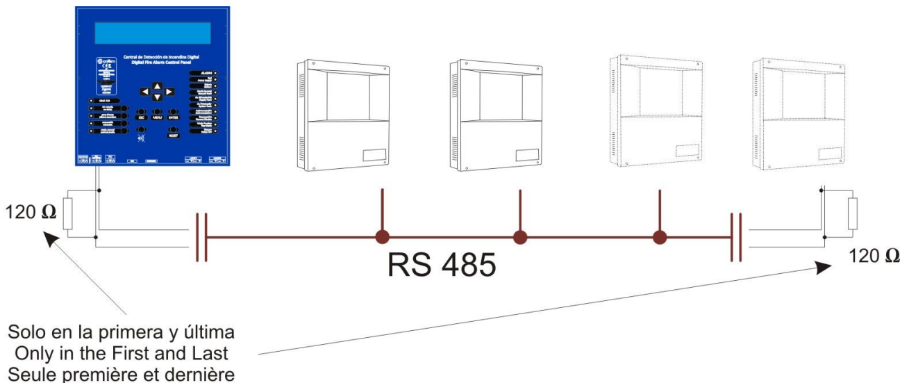
Figure 13. Connexion réseau de centrales
