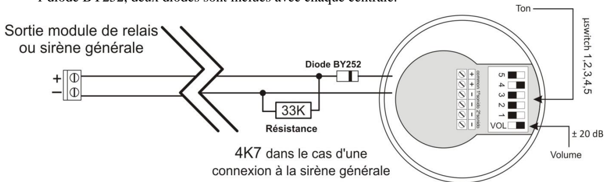
Figure 25. Schéma de raccordement SIR-24B/ SIR-24BL
