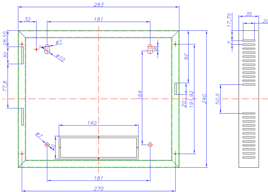
Figure 10. Coffret répétiteur
