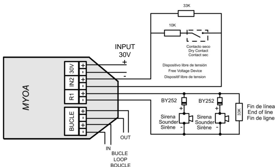
Figure 5. Schéma connexion MYOA/F
