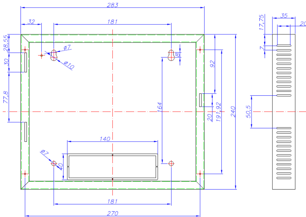
Figura 15. Cofre repetidor
