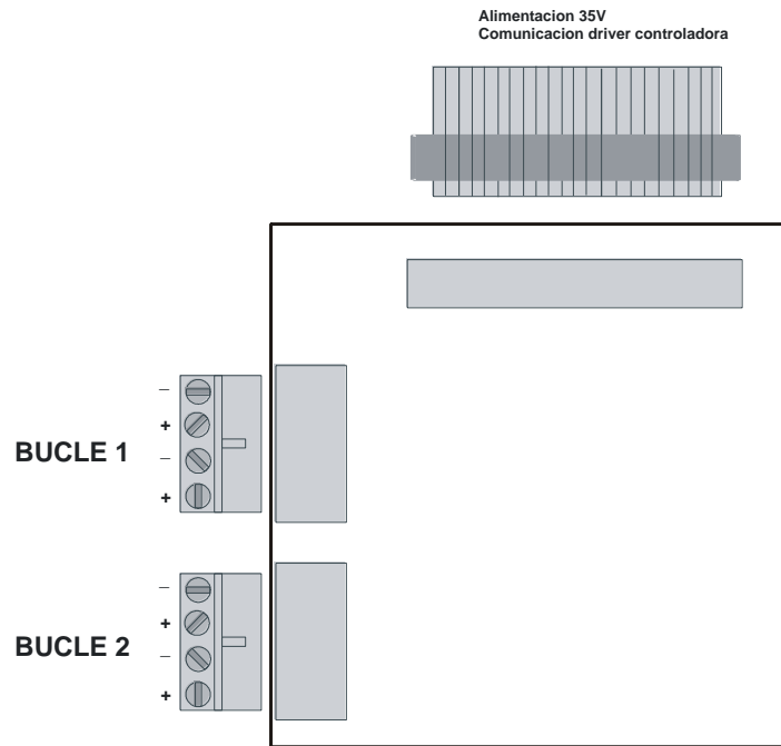
Figura 21. Driver de bucle
