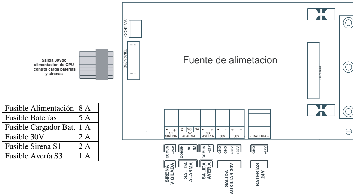
Figura 22. Salidas auxiliares fuente de alimentación
