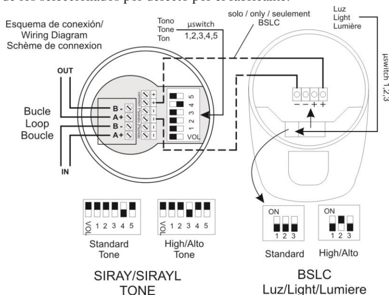
Figura 12. Esquema conexionado SIRAY / SIRAYL / SIRAY+BSLC
