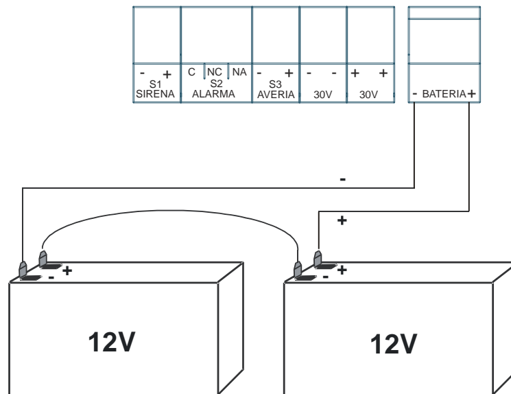
Figura 23. Esquema conexionado baterías
