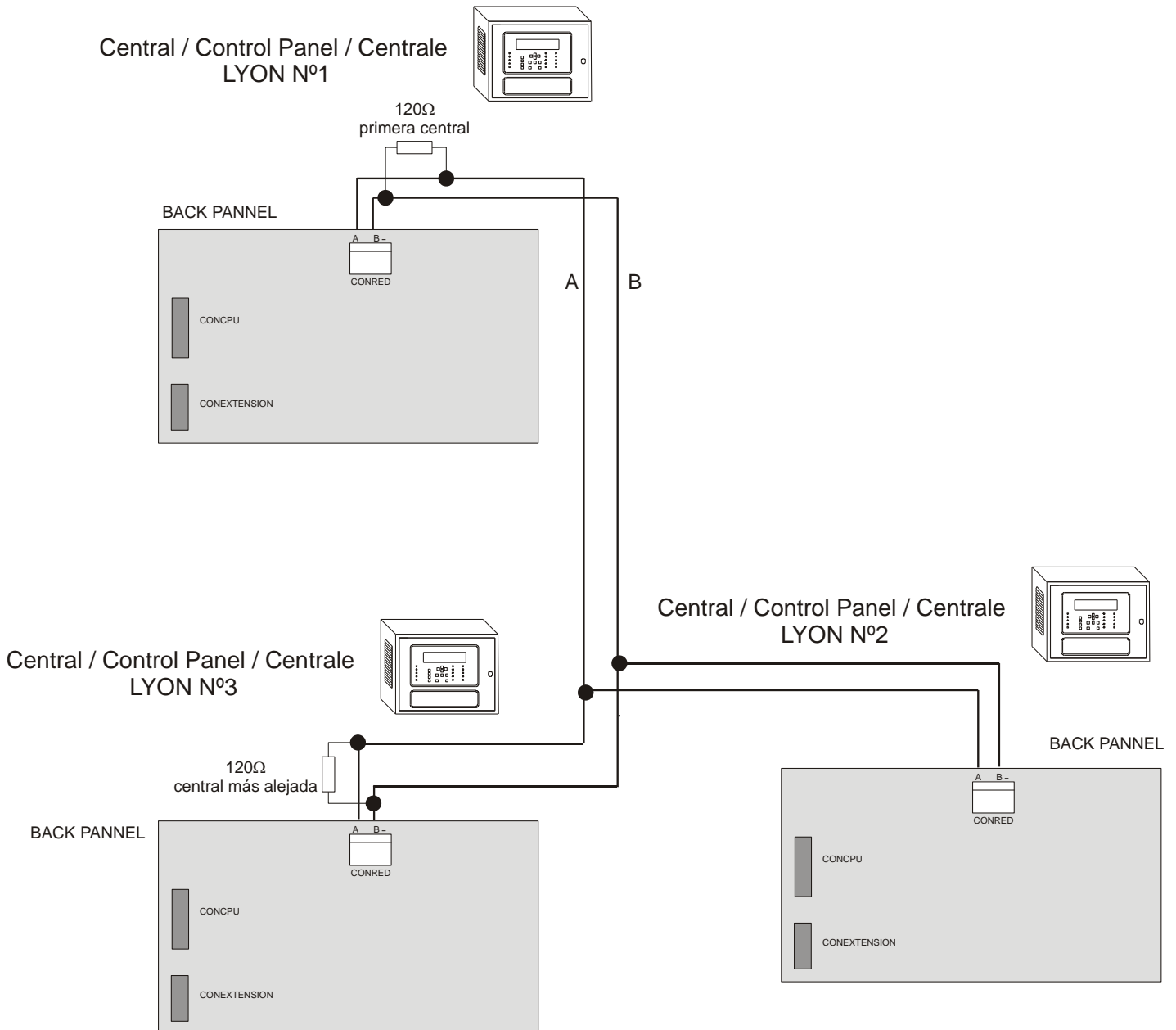
Figura 18. Conexión red de centrales. Max 15
