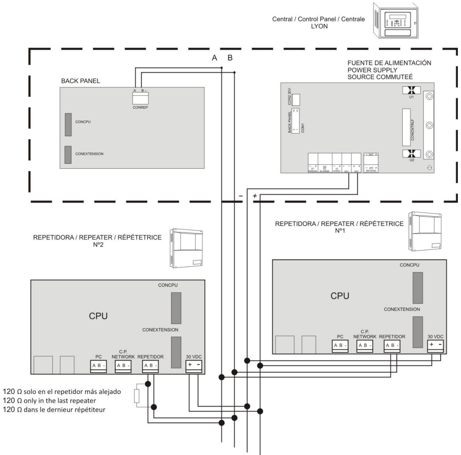
Figura 16. Conexión repetidores. Max 15
