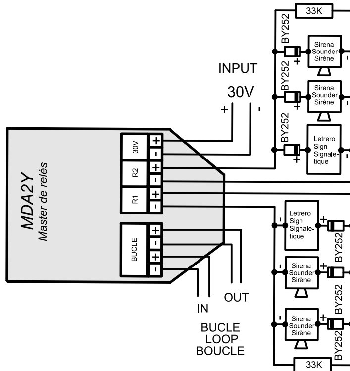
Figura 6. Esquema conexionado MDA2Y
