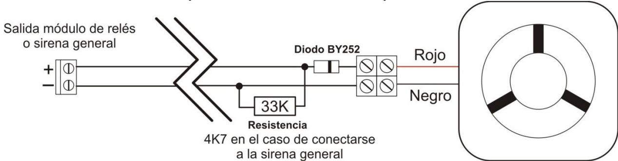
Figura 27. Esquema conexión SIR24F
