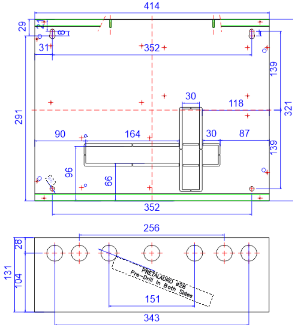
Figura 17. Cofre Lyon
