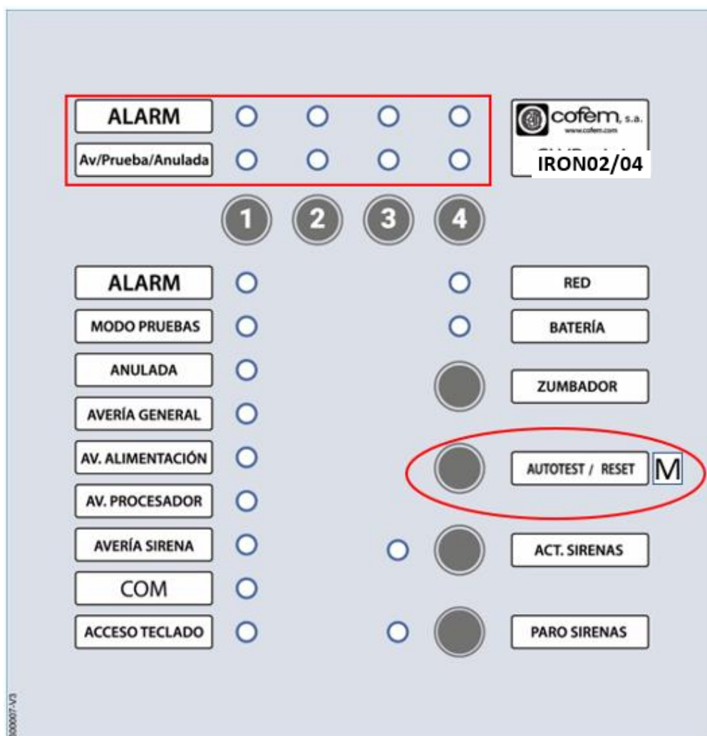
Figura 13: Teclas e Indicadores utilizados en las consultas de versión de firmware y versión de configuración de retardos.
