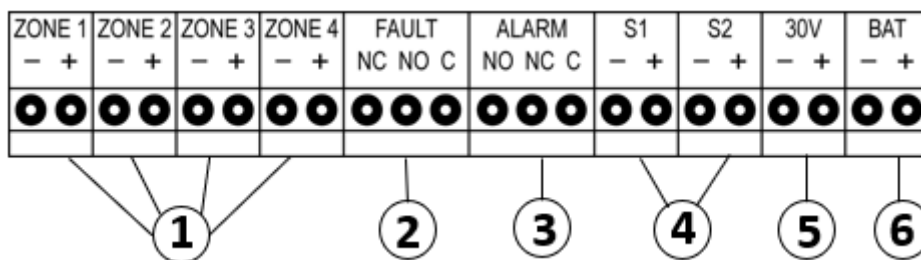
Figura 5: Esquema de los conectores de la central IRON02/04
