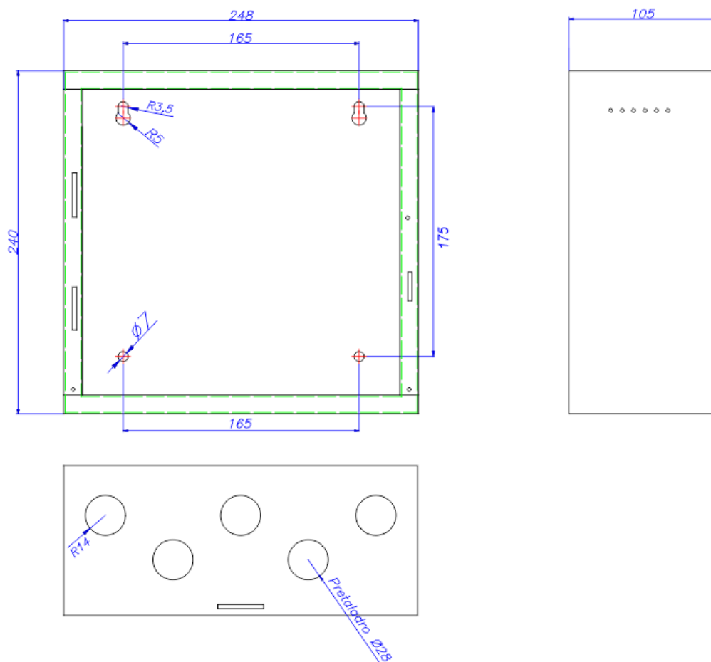
Figure 4: Dimensions coffre et porte de la centrale (mm).
