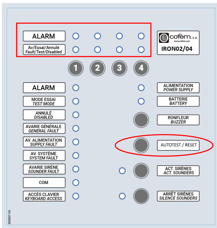
Figure 13: Touches et indicateurs utilisés dans les consultations de version de firmware et de version de configuration de retard.
