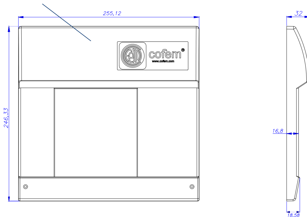
Figure 3 : Schéma coffre et porte de la centrale
