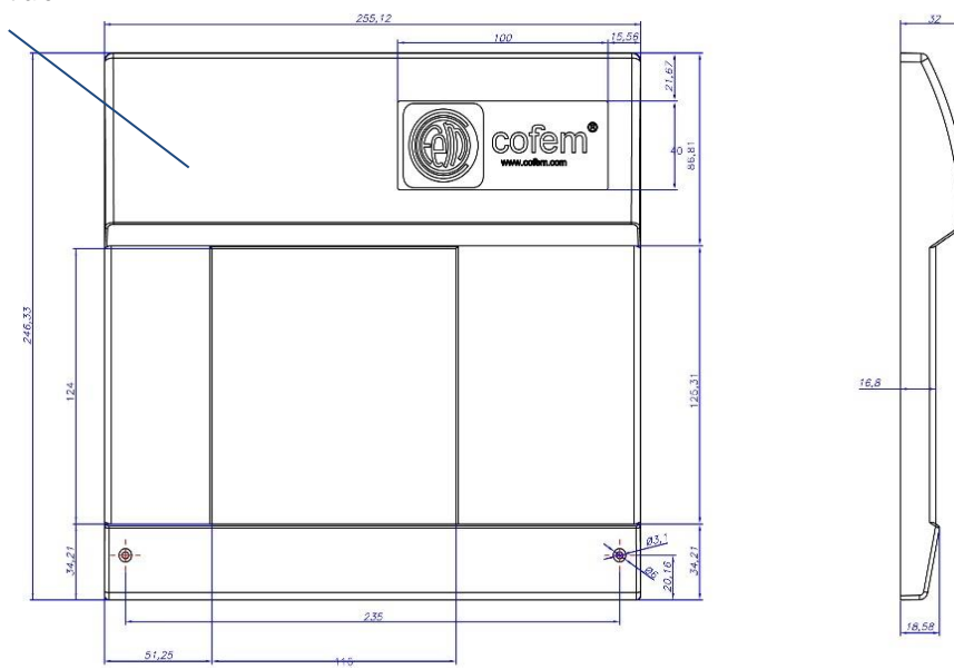
Figure 3 : Schéma coffre et porte de la centrale
