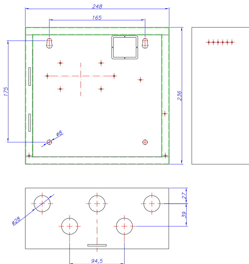
Figura 3: Dimensiones puerta y cofre central (mm).
