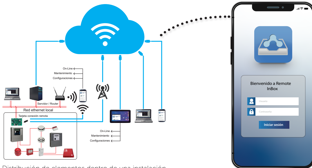
Distribución de elementos dentro de una instalación
