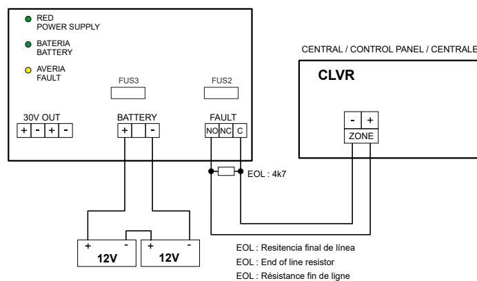
Esquema de conexonado ZAFIRPWS2/5 salida avería
