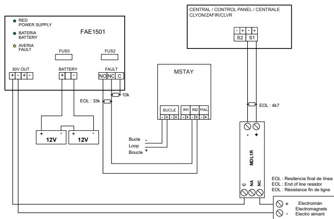
Esquema de conexonado ZAFIRPWS2/5 sistema Algorítmico Direccional
