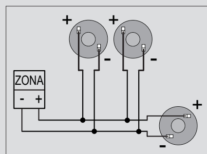
Esquema de conexión
