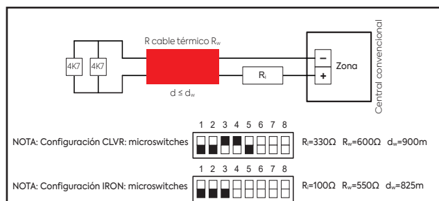
Esquema de conexionado con conexión directa a central convencional
