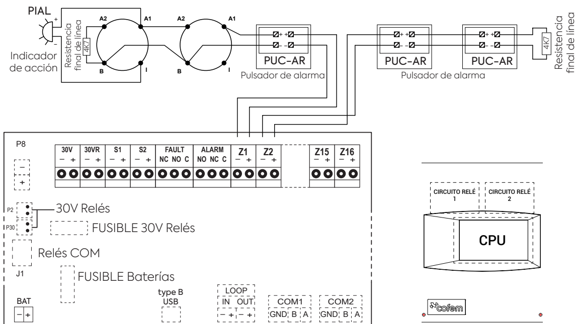
Esquema de conexionado
