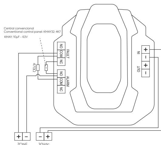
Esquema de conexión DLRC
