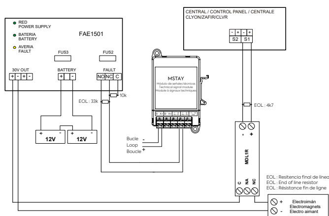
Esquema de conexionado ZAFIRPWS2/5 sistema Algoritmo Direccional
