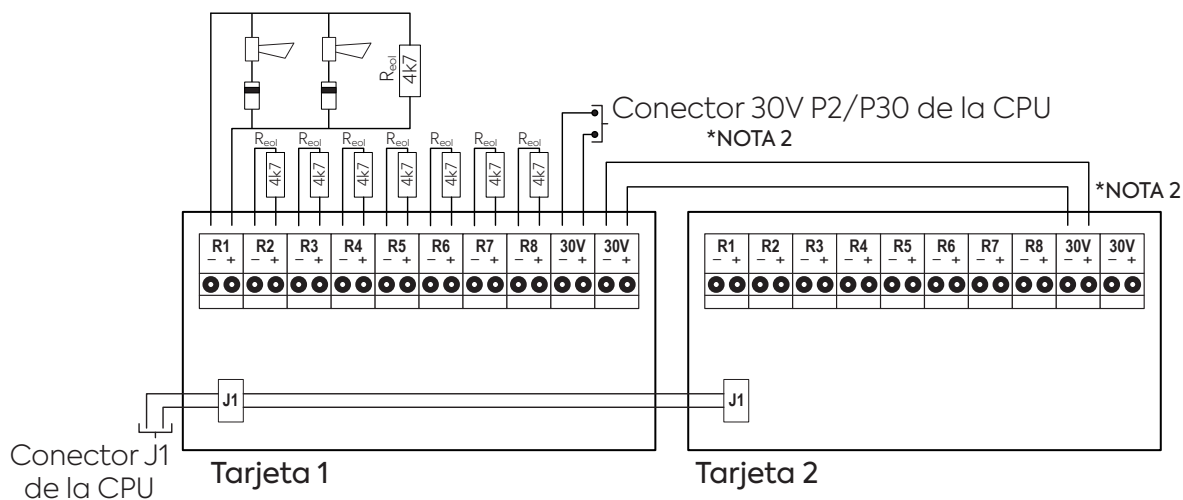
Esquema de conexionado
